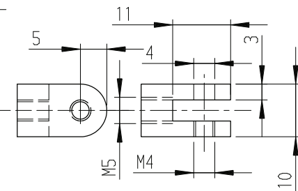
Gabelkopf
