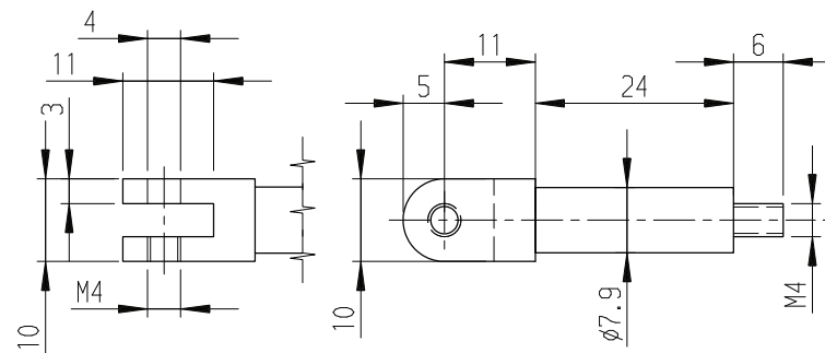
Federbolzen
