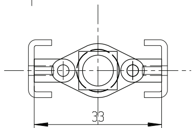
Gleitstange
