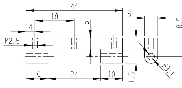
Federbolzen
